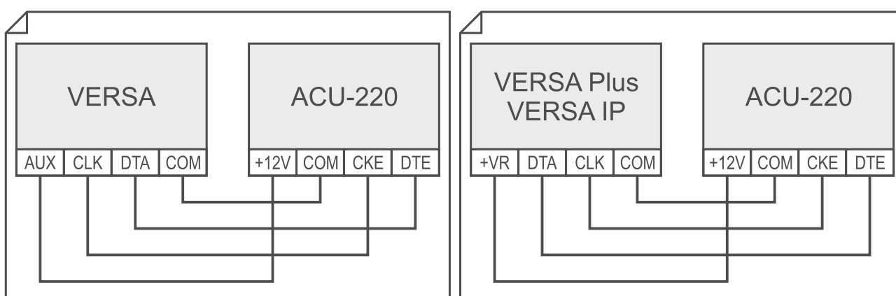
Fig. 8. Manera de conectar el controlador a las centrales de la serie VERSA.
