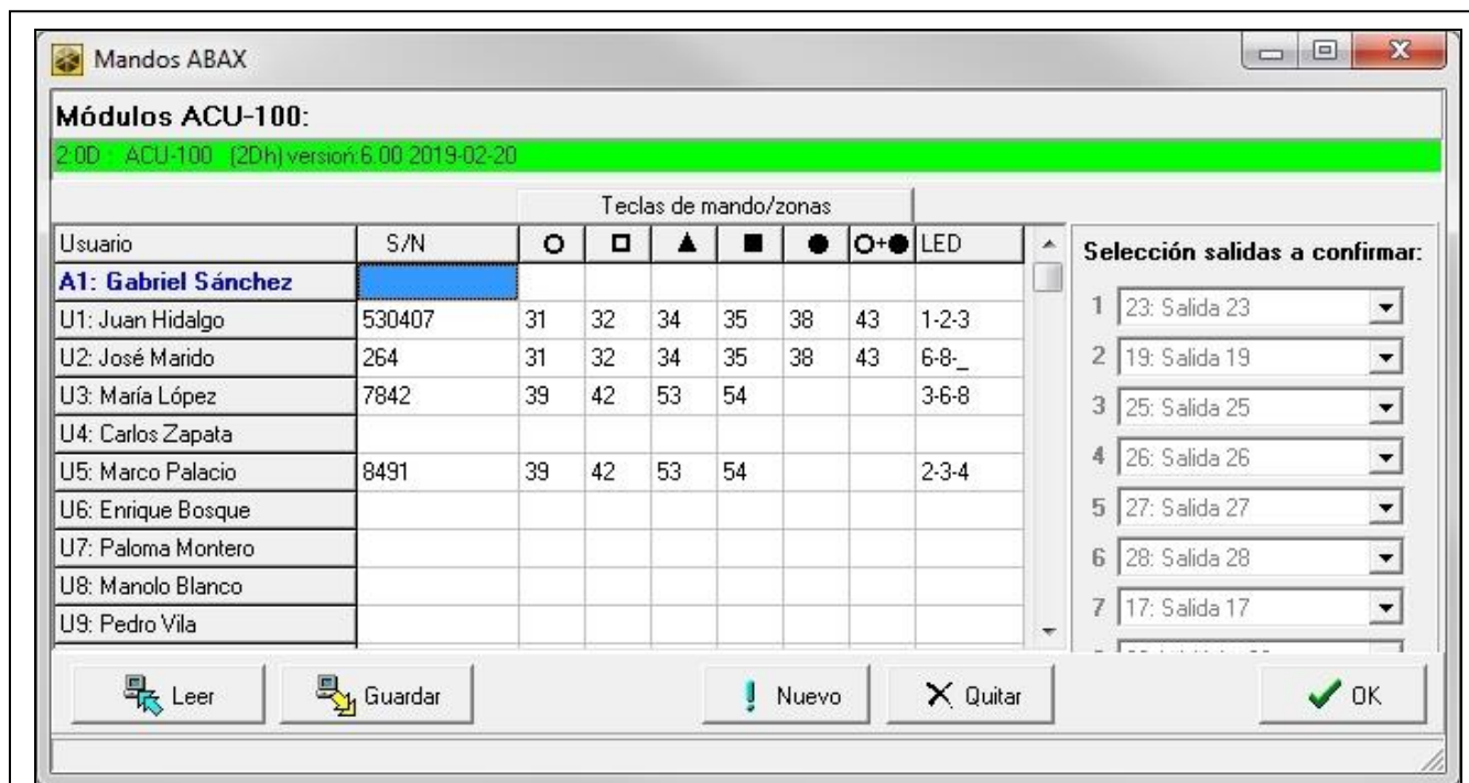
Fig. 28. Programa DLOADX: gestión de mandos a distancia en el sistema INTEGRA.
