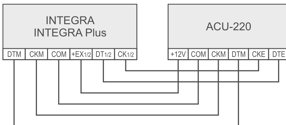
Fig. 7. Manera de conectar el controlador a la central de la serie INTEGRA.
