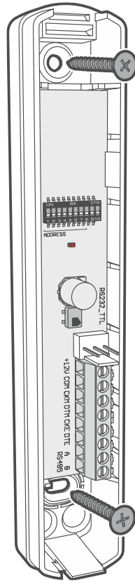
Fig. 6. Montaje de la base de la caja.
