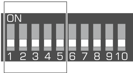
Fig. 3. Interruptor para ajustar la dirección del controlador en el sistema INTEGRA.
